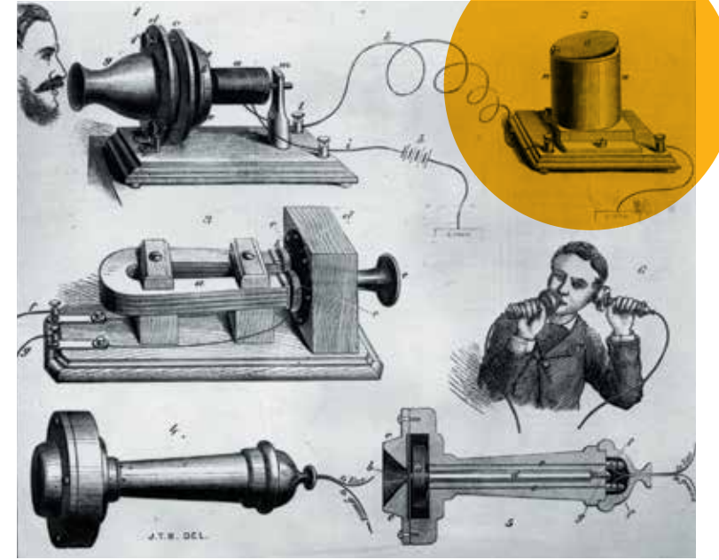
В заявке на патент 1871 года гордо значилось «Телеграфон»
